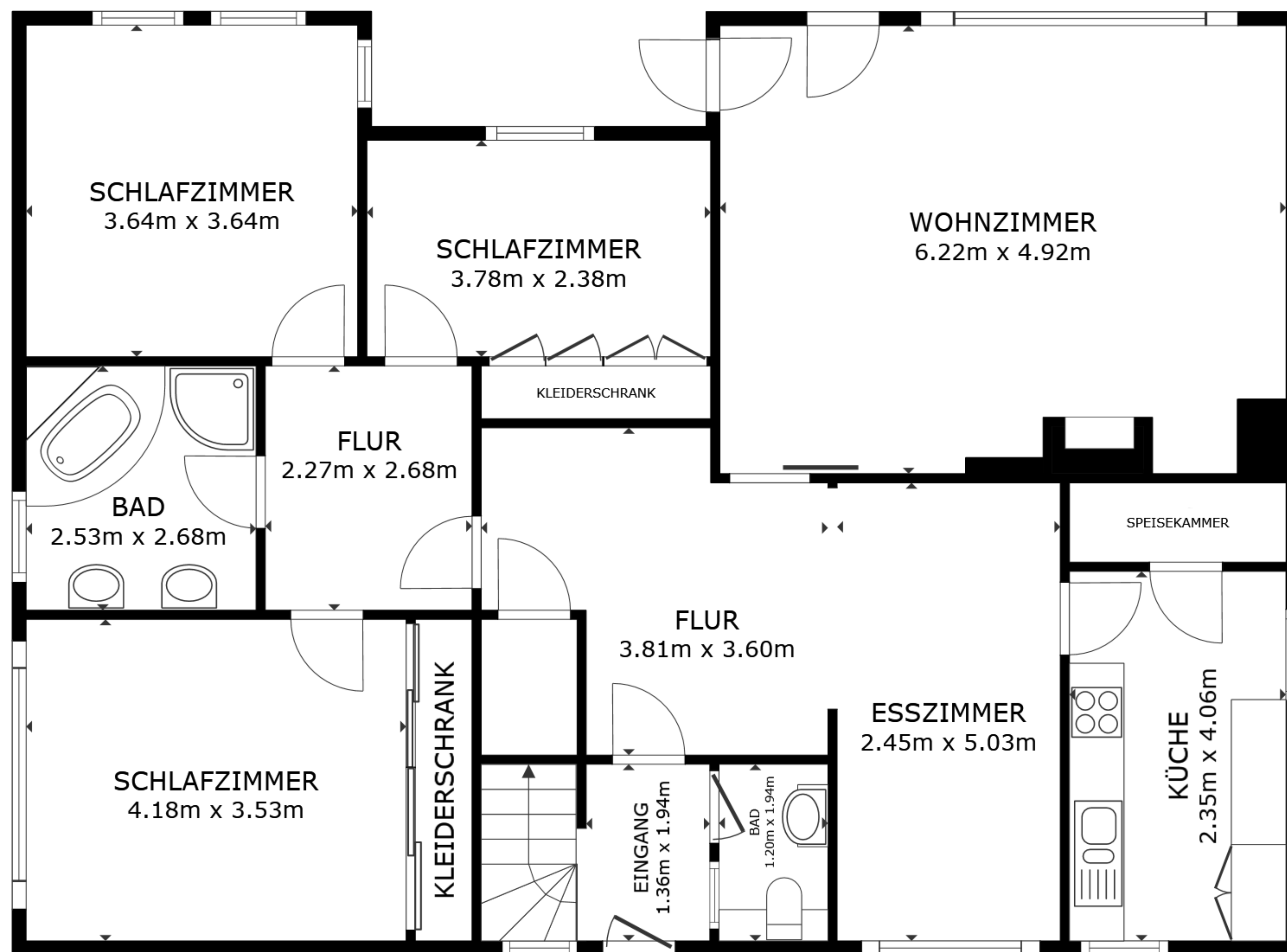
STOCKWERK 1
