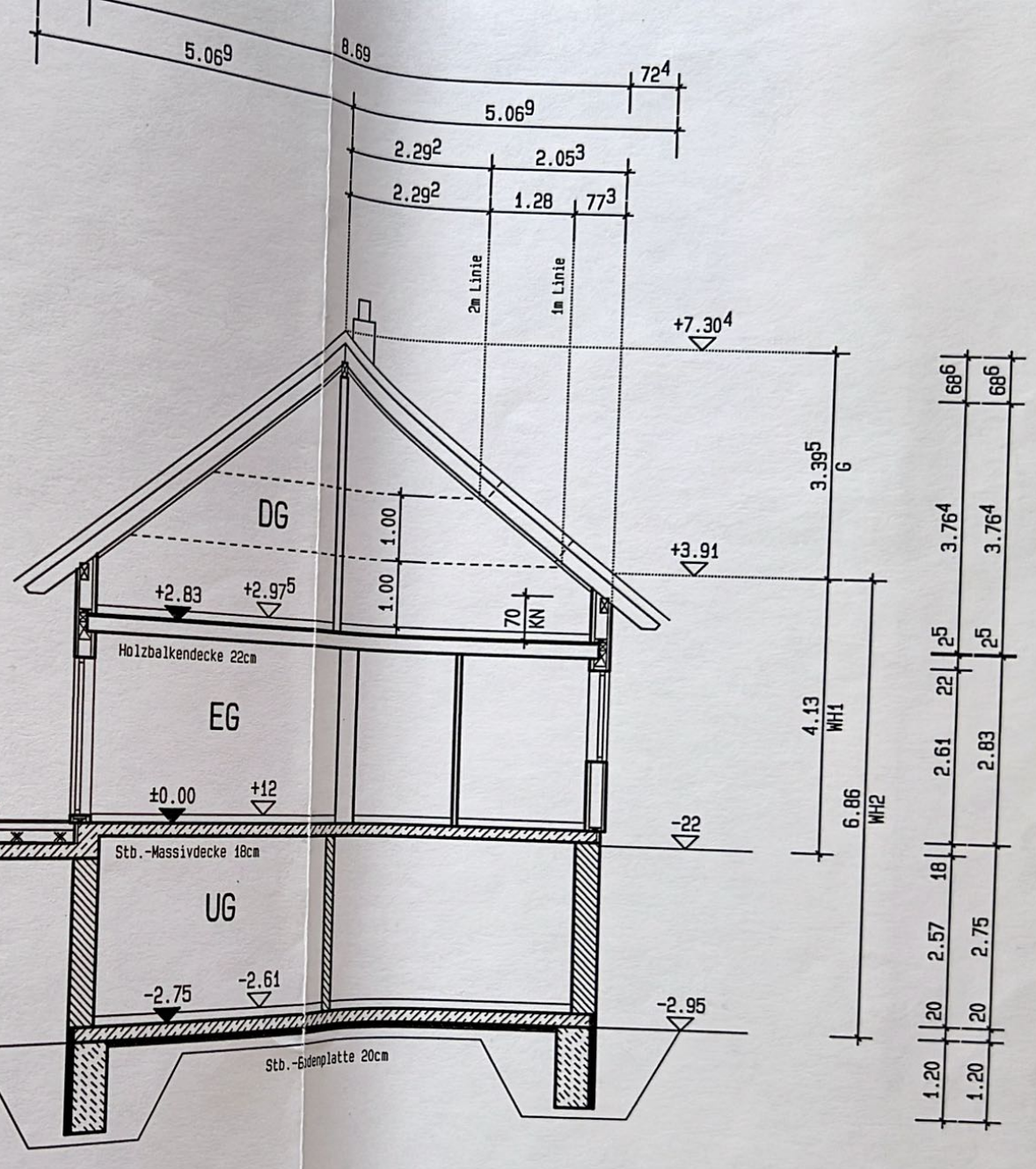
Schnitt Wohnhaus
